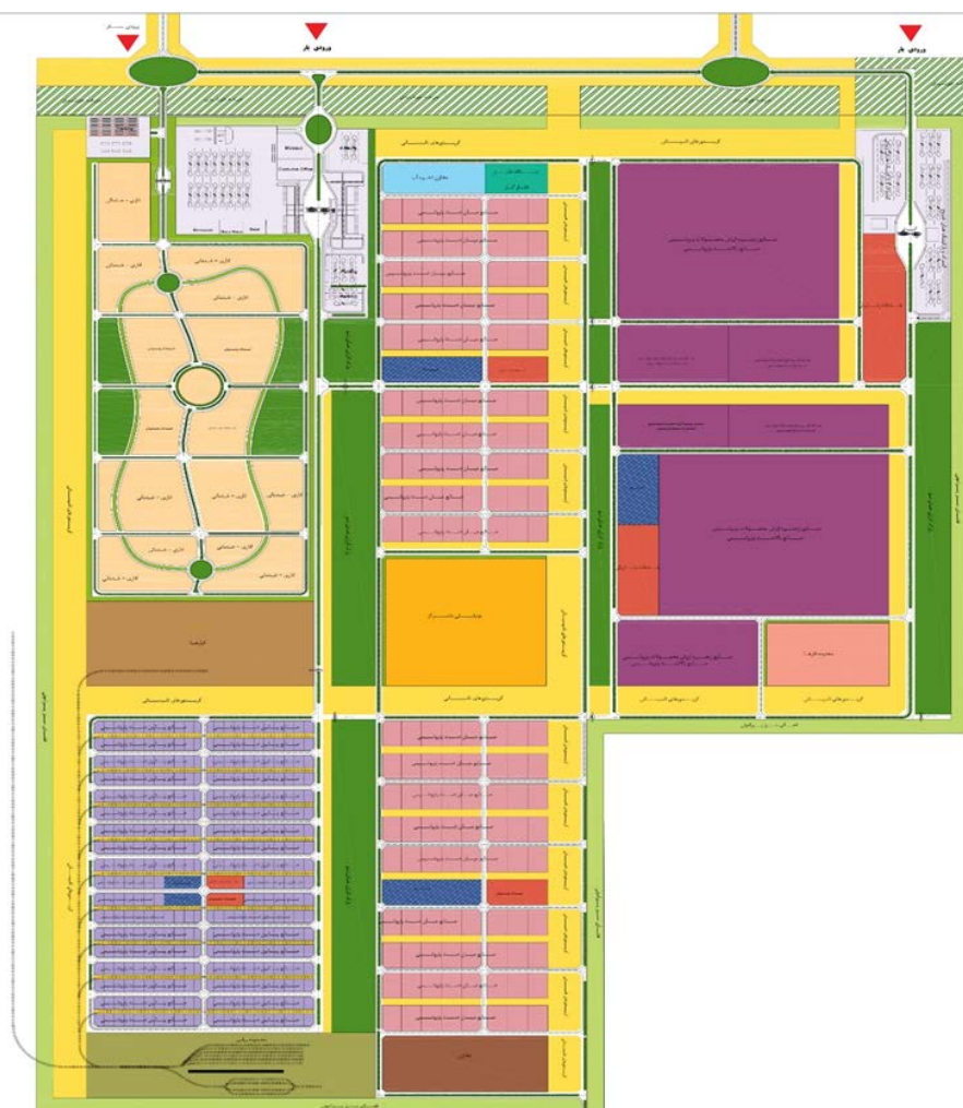
طرح جامع مقدماتی سایت توسعه منطقه ویژه اقتصادی پتروشیمی
