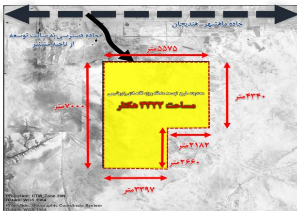
طرح جامع مقدماتی سایت توسعه منطقه ویژه اقتصادی پتروشیمی
